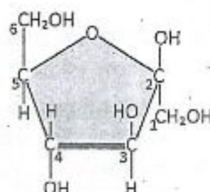
Fructose
