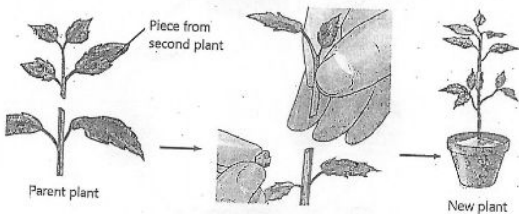
FIGURE 10.13: Grafting
