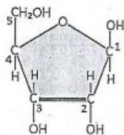
Ribose
