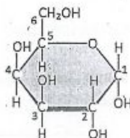
Galactose
