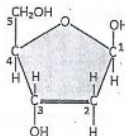
Deoxyribose
